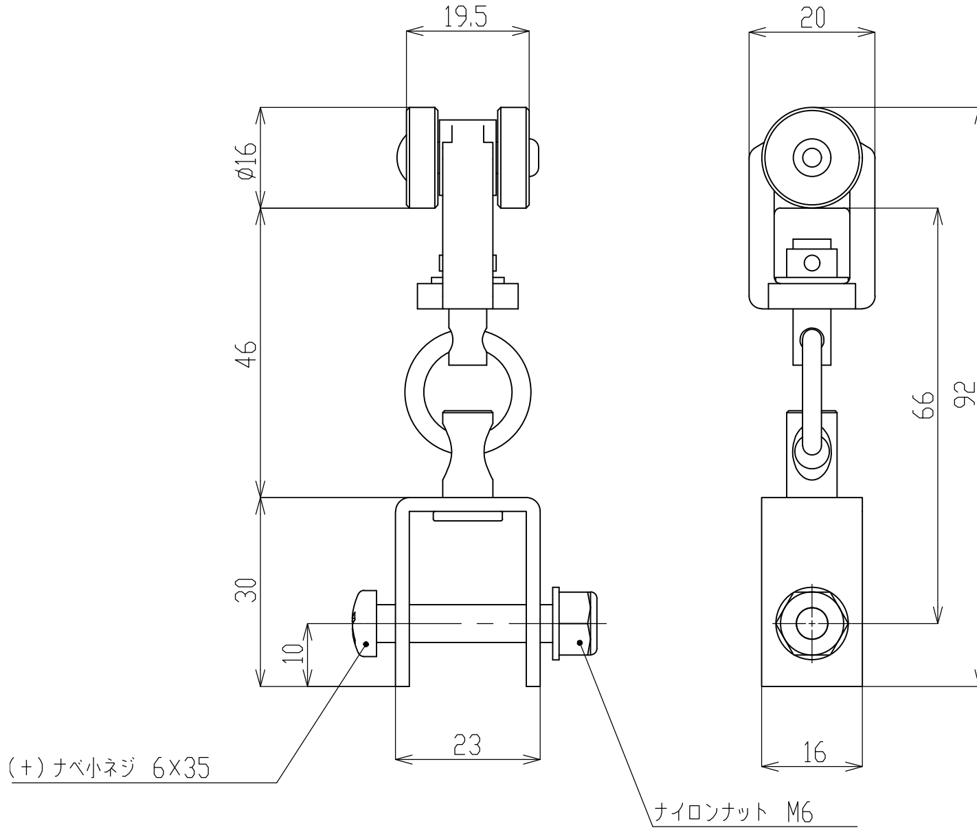
D40間仕切用ランナーN (15T28N)
