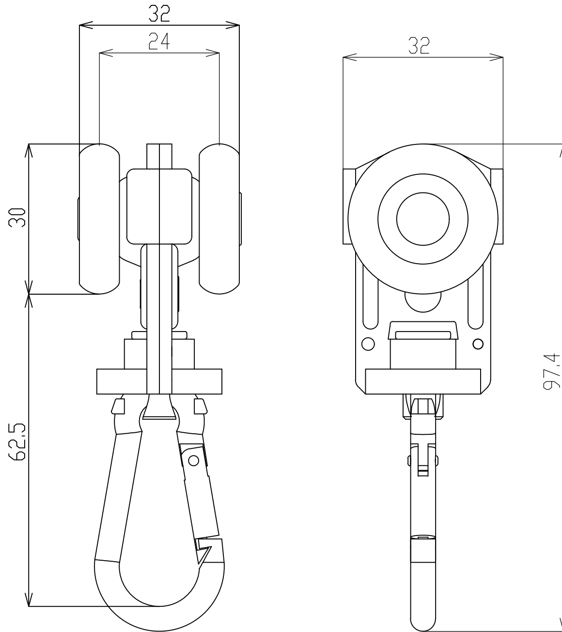
SGベアリング入ワンタッチランナーDN (27T29DN)
