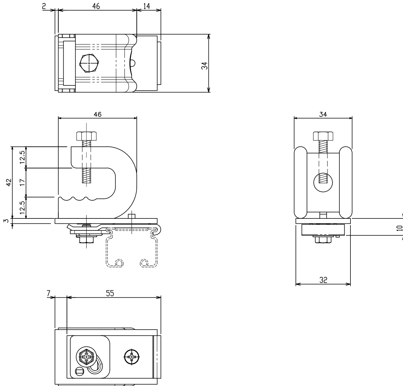
D30クリップ付き天井ブラケットANタイプ (12Y17N)
