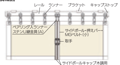
両開構成図
