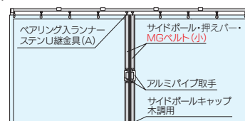
片開構成図
