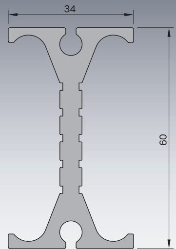
■キャリアレール断面図 (mm)
