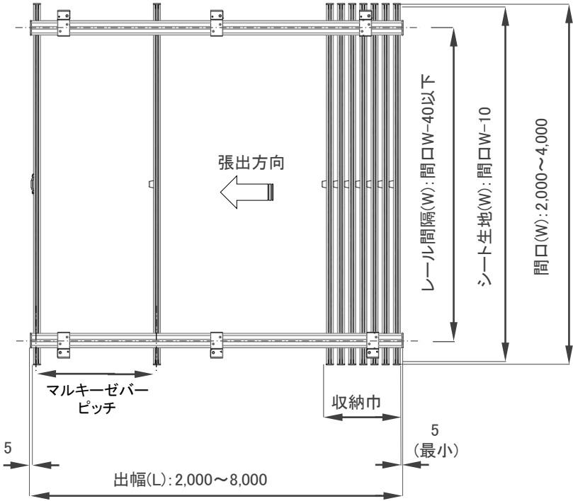
[側面図]
