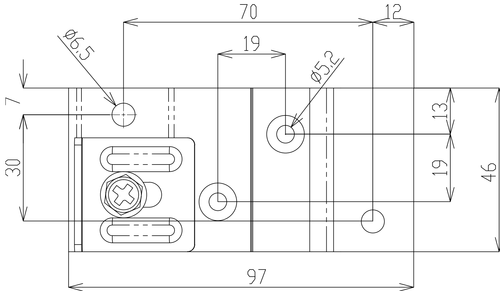
HG天井後付Sブラケット (24T52)
