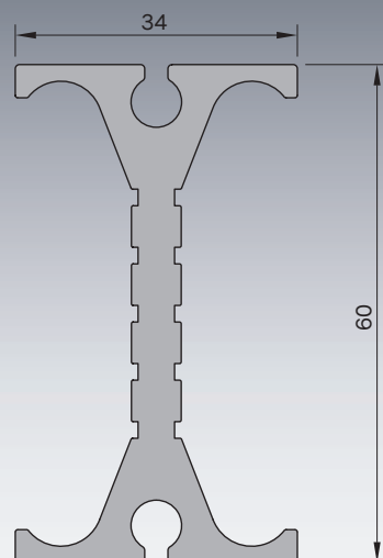
■ キャリーレール断面図 (mm)
