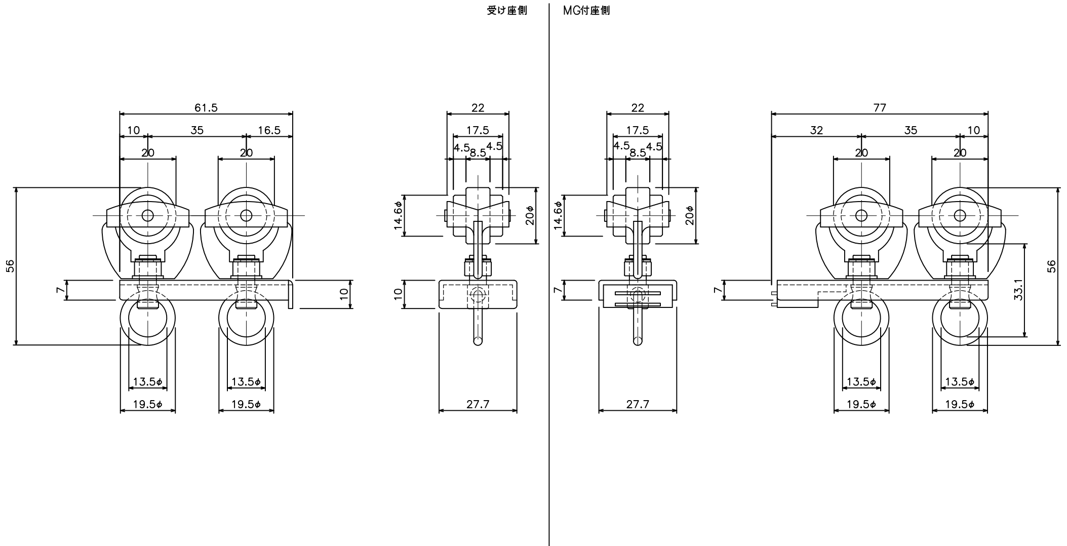
D40 マグネットランナー(両開)ステージランナー(15Y22)
