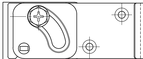
D40 ステンクリップ付天井ブラケット (Aタイプ) (25Y15)
