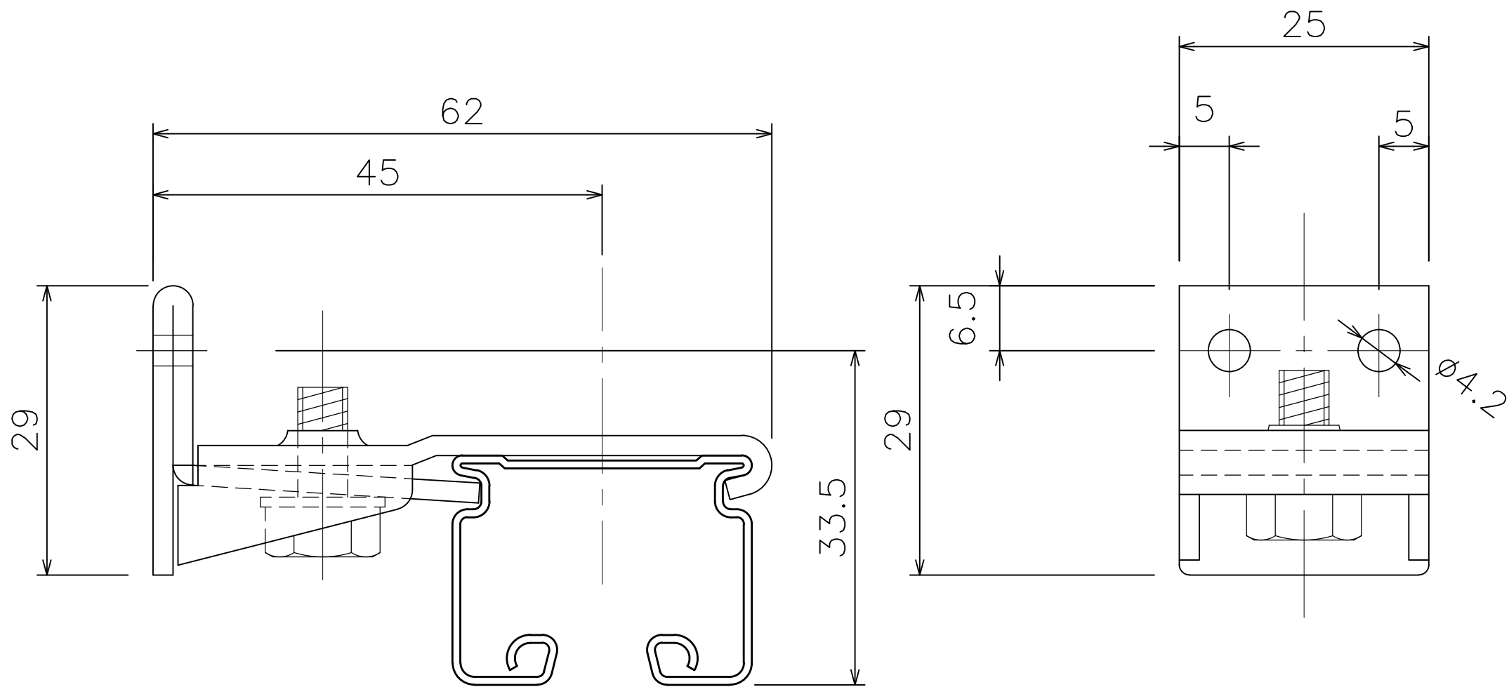
D30 Sブラケット (12T41)
