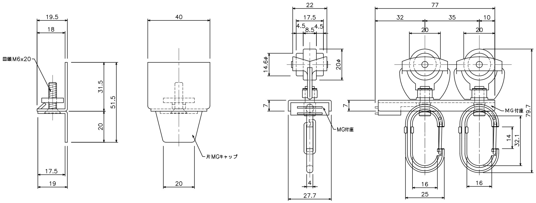
D40片マグネットランナー(片開)ワンタッチランナー S(15Y34)
