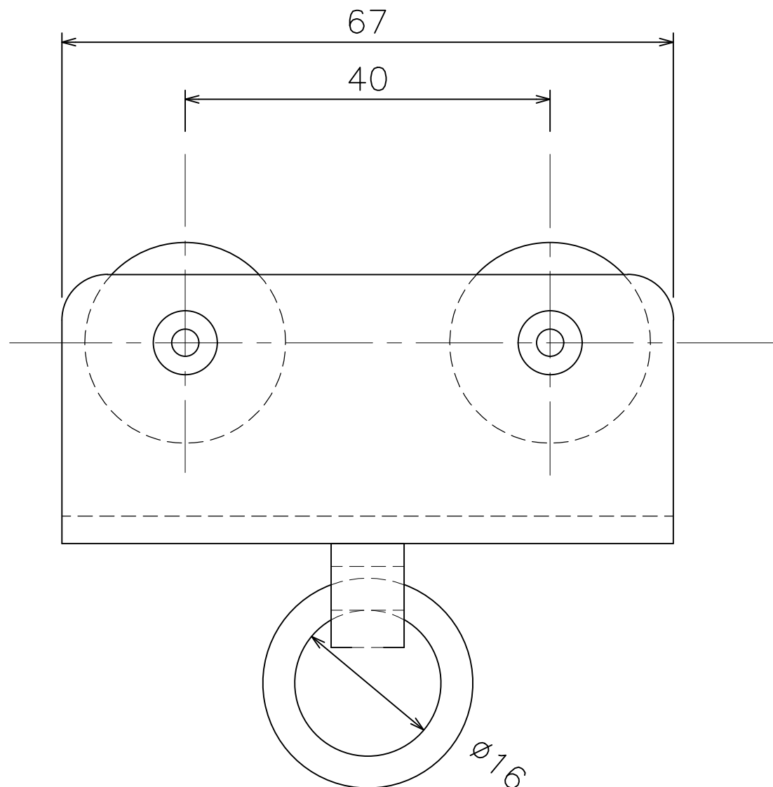
ベンダーベアリング入複車ランナー (19T29)
