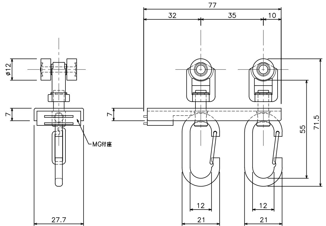
D30片マグネットランナー(片開)ワンタッチランナー (12Y33)
