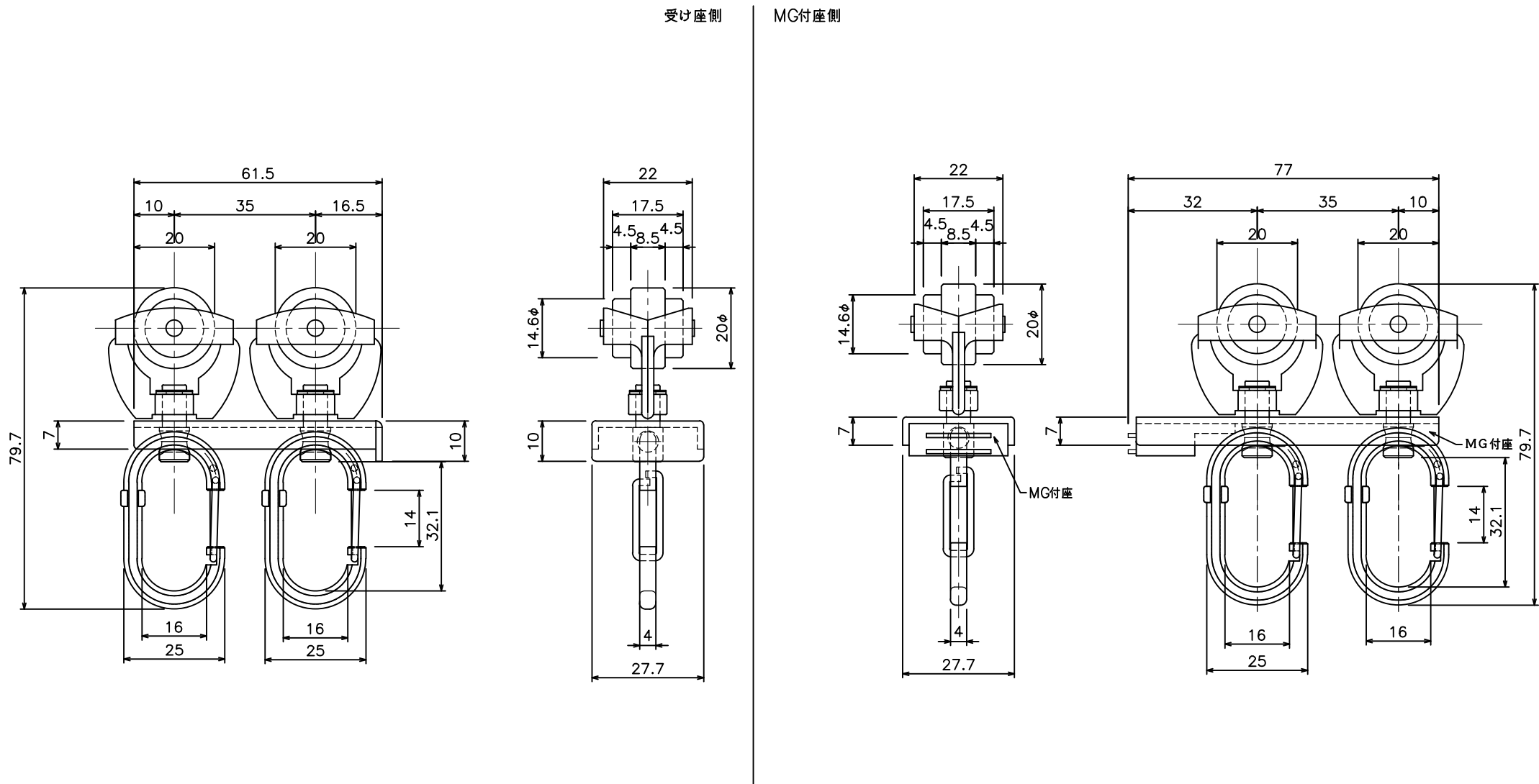
D40 マグネットランナー(両開)ワンタッチランナーS(15Y24)
