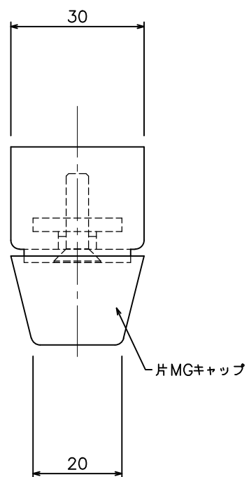
D30片マグネットランナー(片開)通常ランナー (12Y31)
