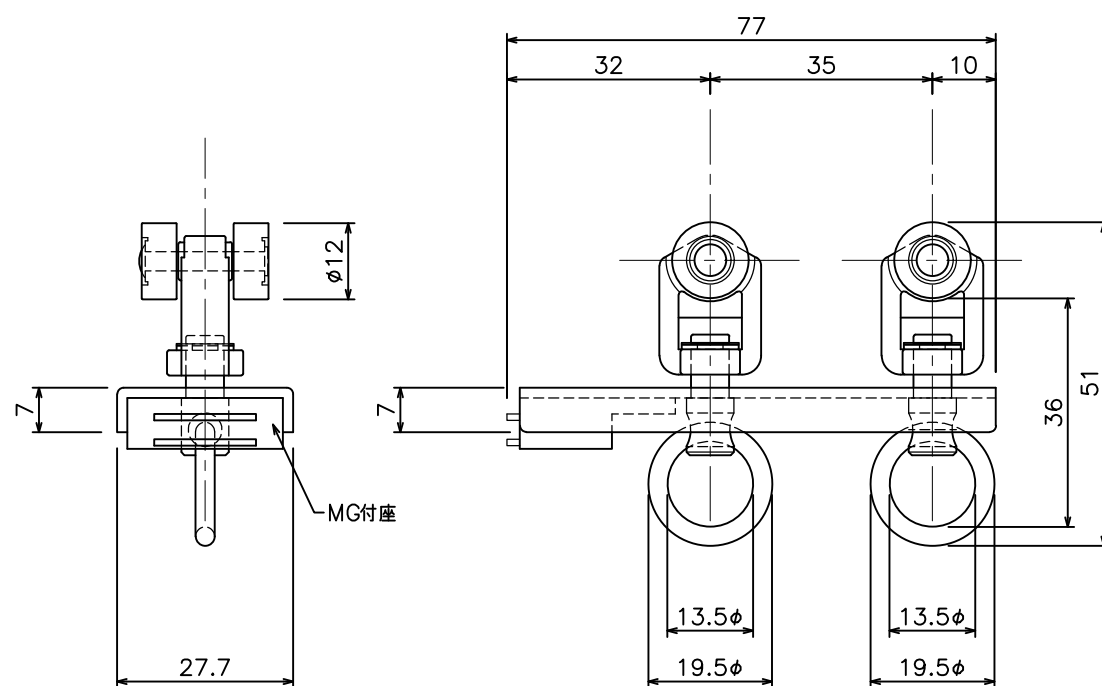
D30片マグネットランナー(片開)通常ランナー (12Y31)
