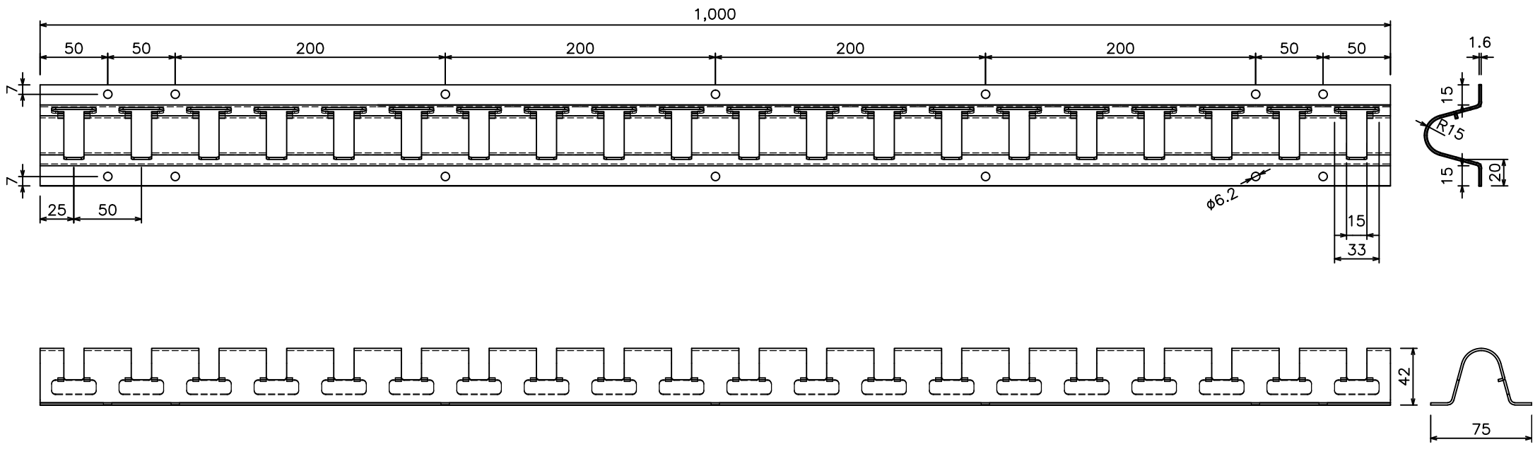
のれんシートフレーム【Bタイプ】寸法図スケール(72B11)
