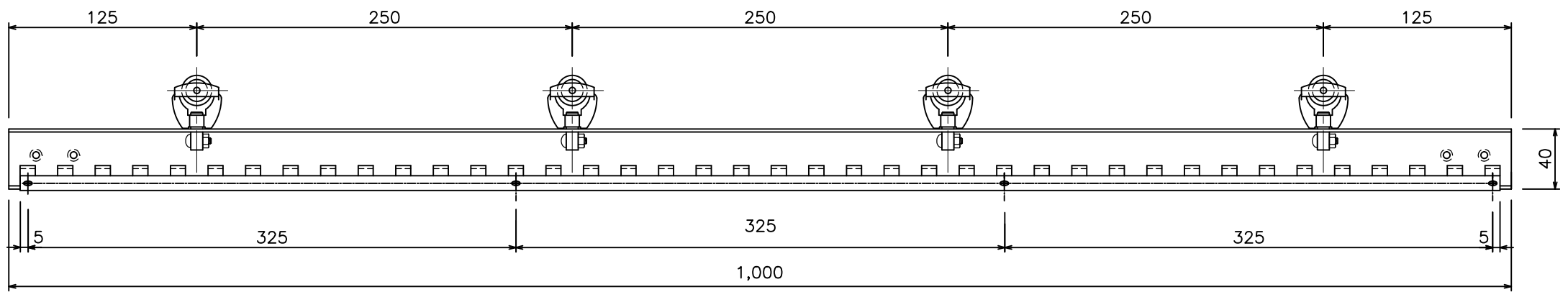
のれんシートフレーム【Aタイプ】可動式 roller 寸法図 (72A62)
