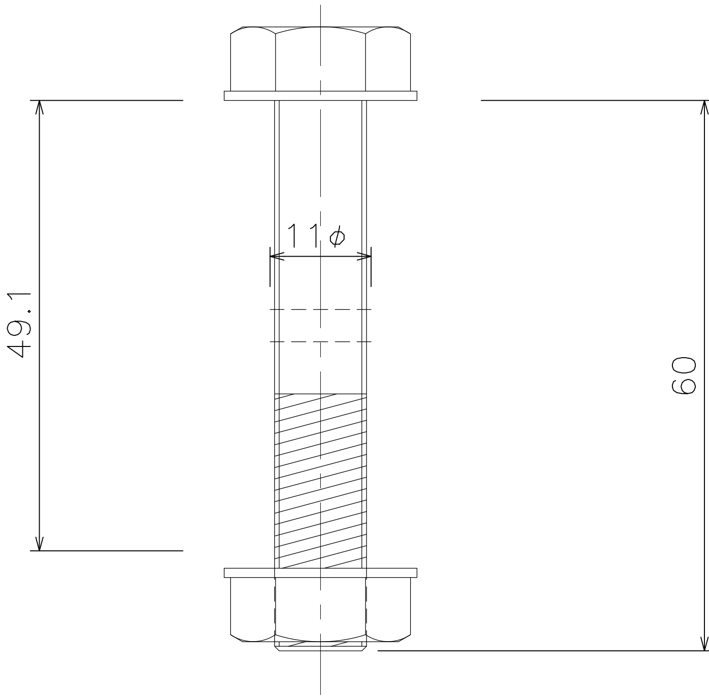
開閉シート ストッパー (26T31)
