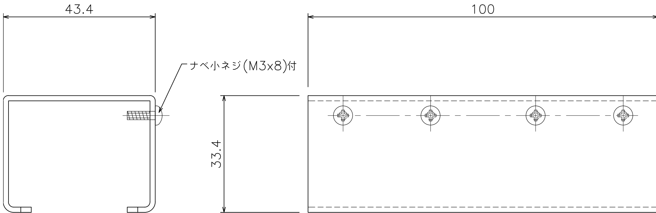
D40 ステン継カバー (25T 62)
