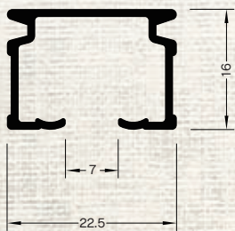
アルミ押出型材
