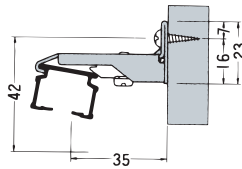
Sブラケット
