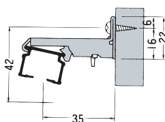
完全ワンタッチSブラケット
