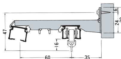
Wブラケット
