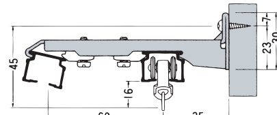
Wブラケット
