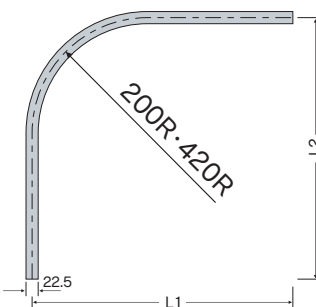
●別注カーブレール寸法図 (mm)
