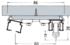
天井Wブラケット
