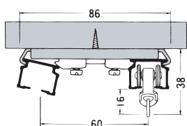
天井Wブラケット
