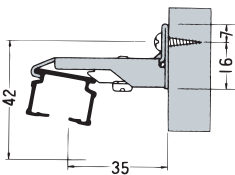
Sブラケット
