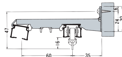
完全ワンタッチWブラケット
