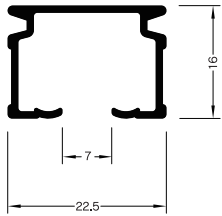
アルミ押出型材
