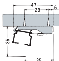
天井Sブラケット
