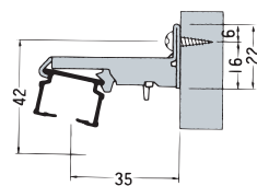
完全ワンタッチSブラケット
