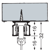
天井直付
