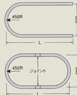
●U・Oカーブレール寸法図 (mm)
