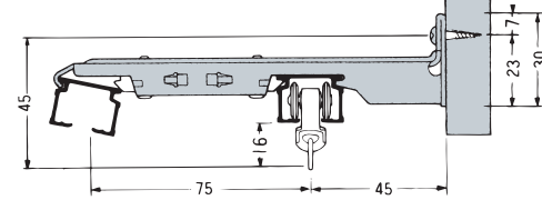
ロングWブラケット
