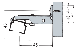
ロングSブラケット
