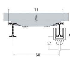
天井Wブラケット
