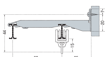
Wブラケット
