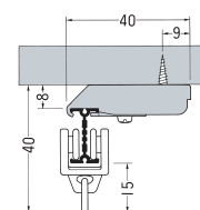
ワンタッチ天井Sブラケット
