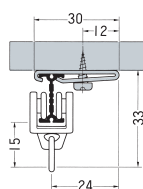
天井Sブラケット
