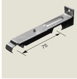
CロングWブラケット (1T46) (住宅公園AI-911C1型用)
