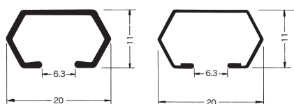
アルミ押出型材
