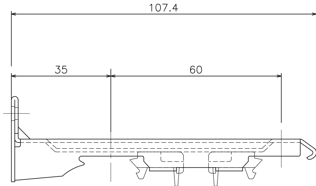
D25 完全ワンタッチWブラケット (9T42)
