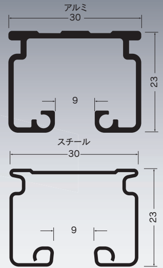
D30レール断面図 (mm)
