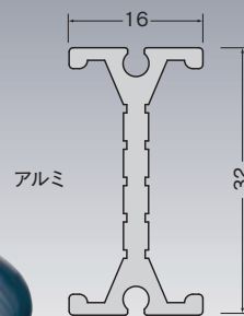
ベンダーレール 断面図 (mm)
