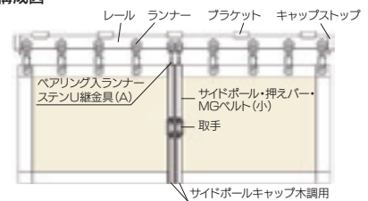
両開構成図
