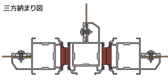
三方納まり図
