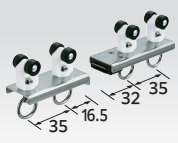
D30マグネットランナー(両開) 通常ランナータイプ
