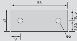
吊棒天井付面 寸法図
