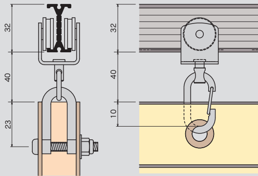
ベアリング入ランナー U継金具
