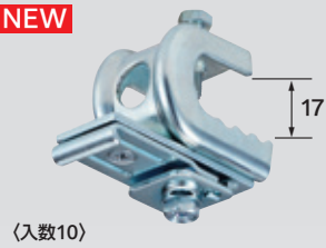
ANタイプ 12Y17N スチール/ユニクロ ¥1,300/個 適合フランジ厚 3~16mm
