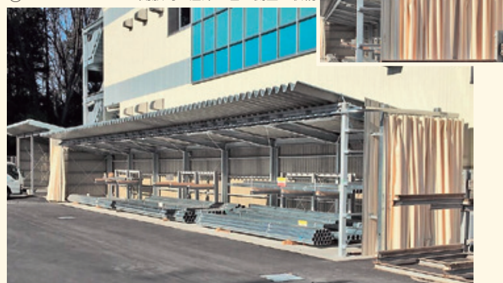
レールを90°曲加工、 シート開放時に倉庫左右の側面に収納
