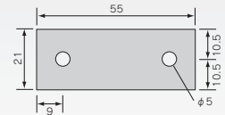
吊棒天井付面寸法図
