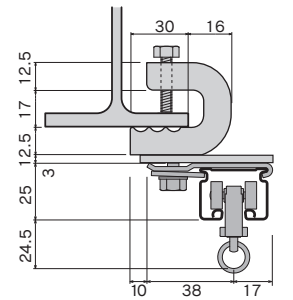
鋼材から持ち出し
