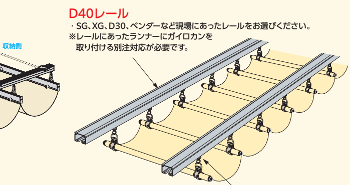
D40ランナーワイロカン付 ・レールに合わせその他のランナーでも別注対応が可能です。
