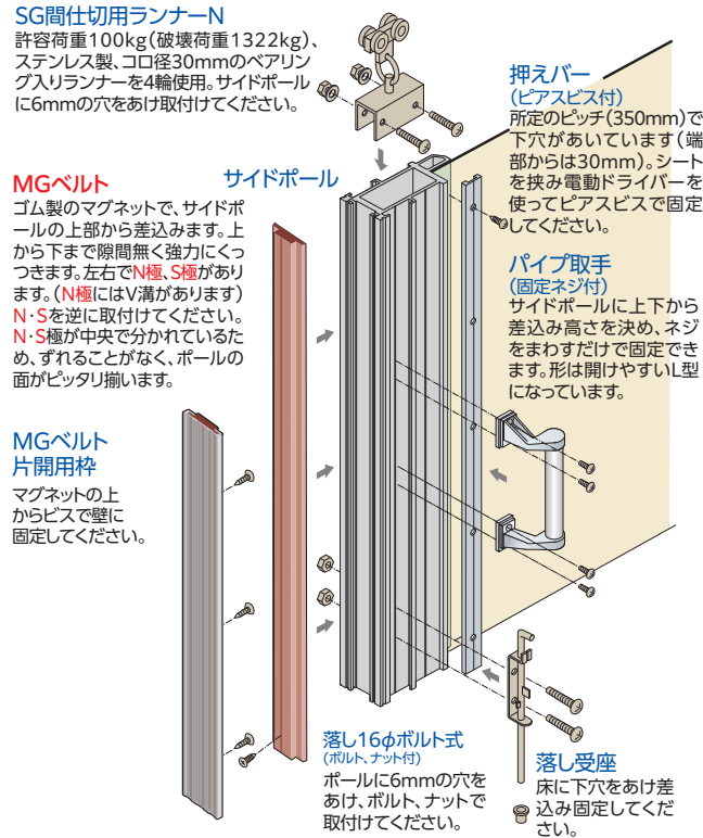
SGランナーN・SGステンU継金具
