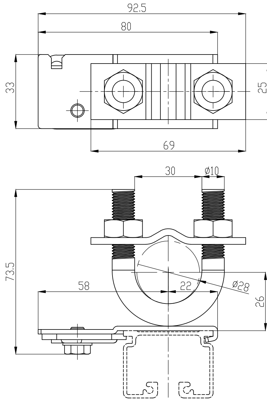
D40Uボルト付天井ブラケットN 28φ用 (15Y01N)
