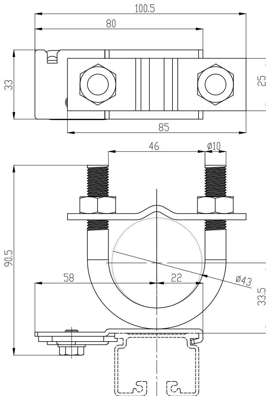
D40Uボルト付天井ブラケットN 43φ用 (15Y03N)
