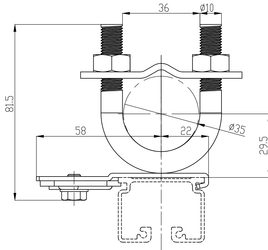
D40Uボルト付天井ブラケットN 35φ用 (15Y02N)
