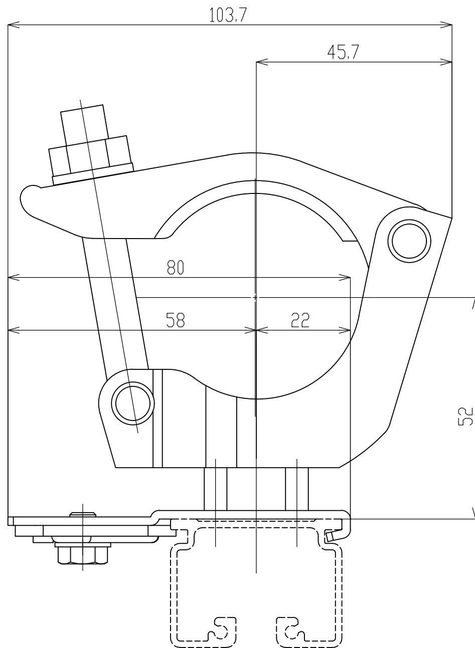
D40クランプ付天井SブラケットN (15Y20N)
