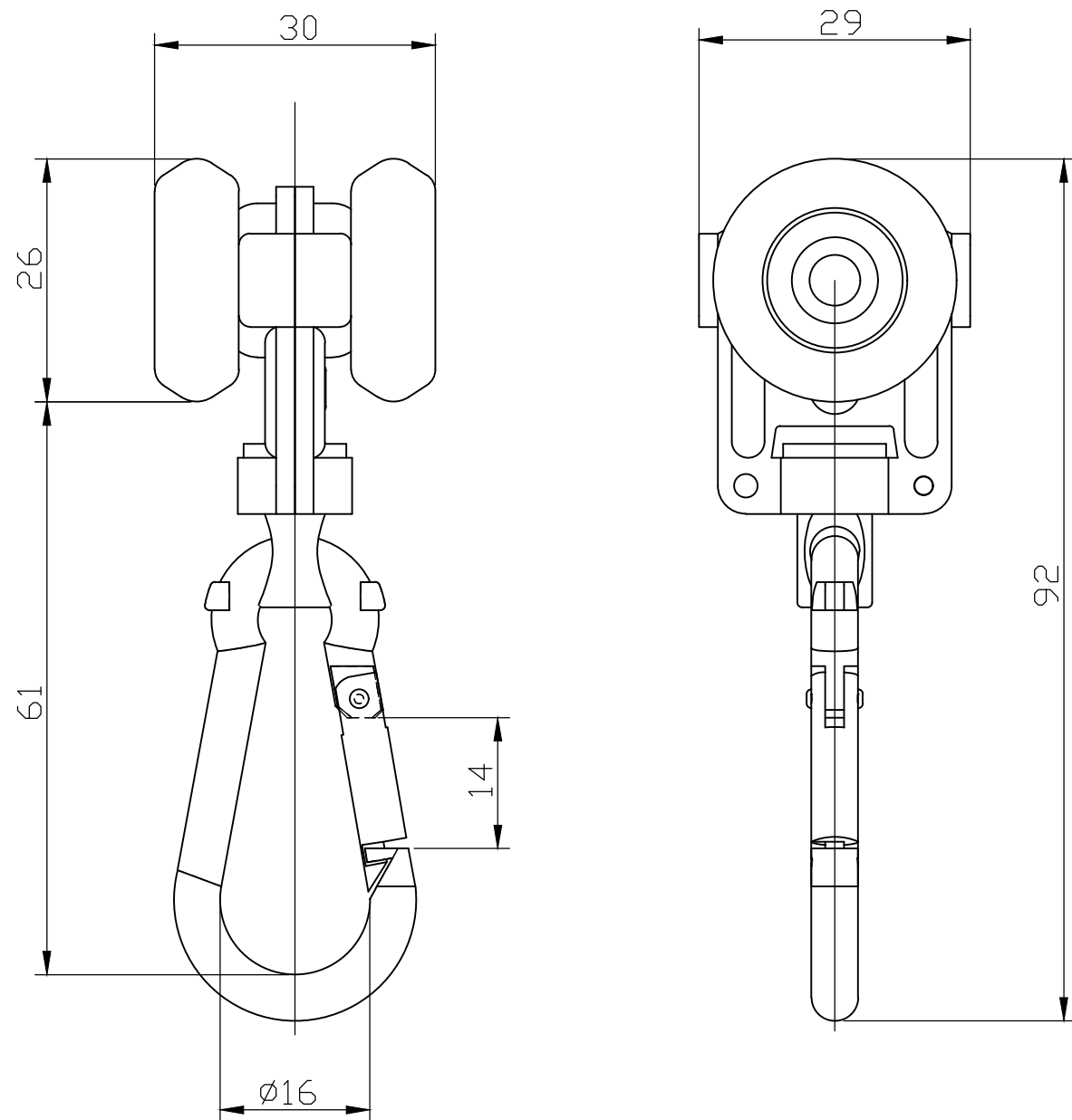
XGステンベアリング入ワンタッチランナーD (29T22D)
