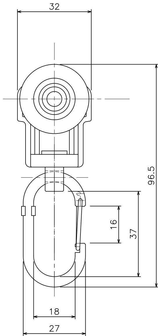
SG ベアリング入ワンタッチランナーN (27T29)
