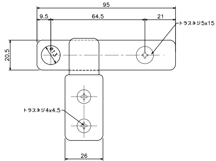
間仕切ロック両開ステン (90T36)
