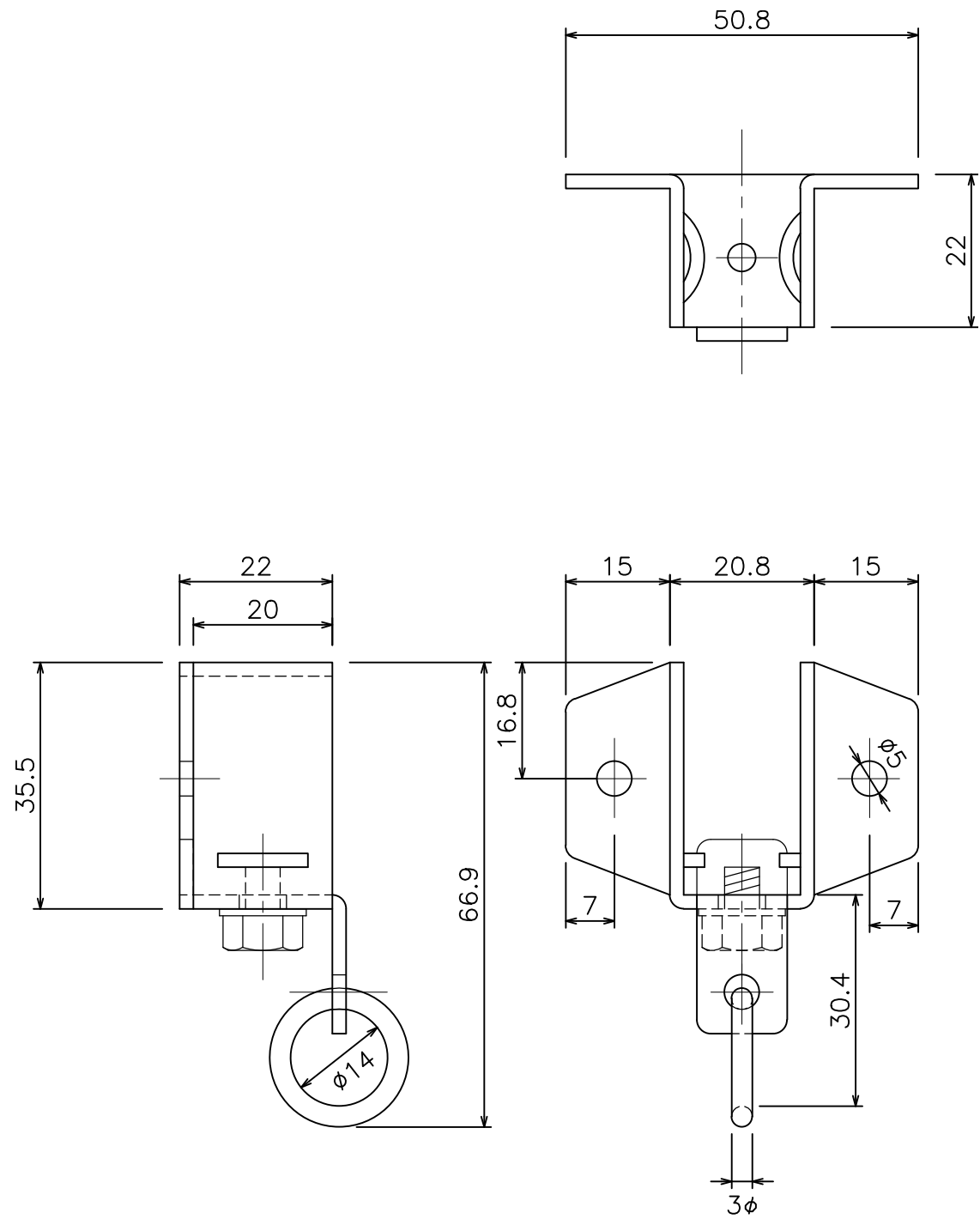
ベンダー 壁付ソケット (19T36)
