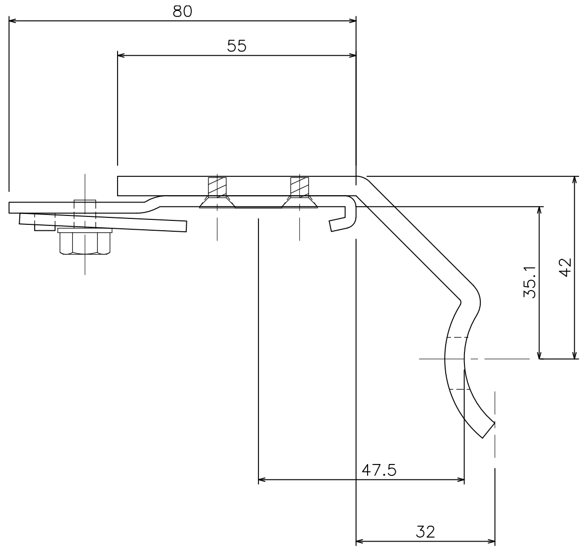
D40 パイプ用ブラケット 38φ (15Y42)
