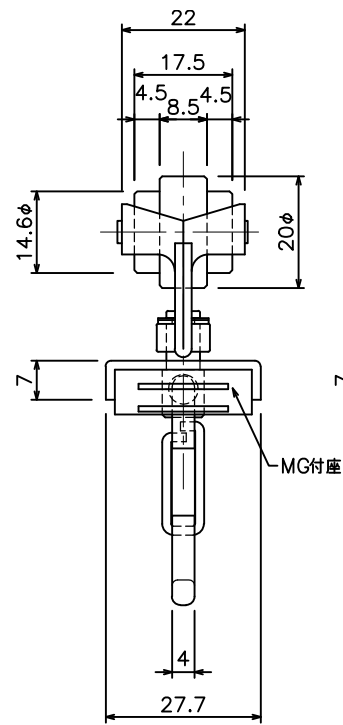
D40片マグネットランナー(片開)ワンタッチランナー S(15Y34)
