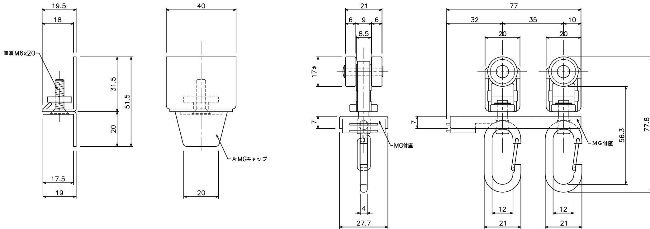
D40片マグネットランナー(片開)ワンタッチランナーA (15Y33)
