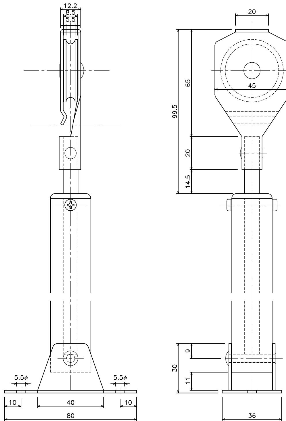
D40 紐止プーリー (15T74)
