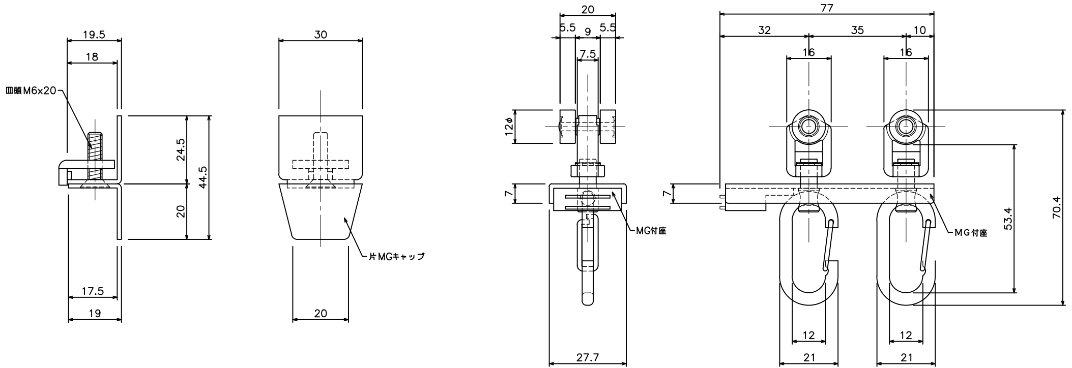
D30 片マグネットランナー(片開)ワンタッチランナー(12Y33)
