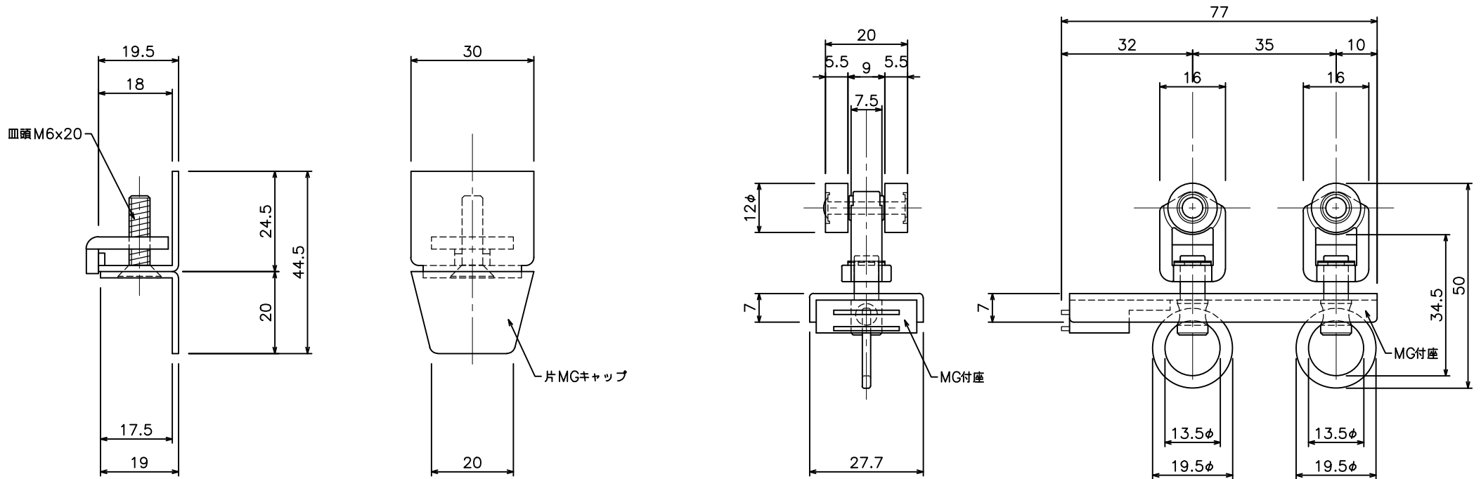
D30 片マグネットランナー(片開)通常ランナー(12Y31)
