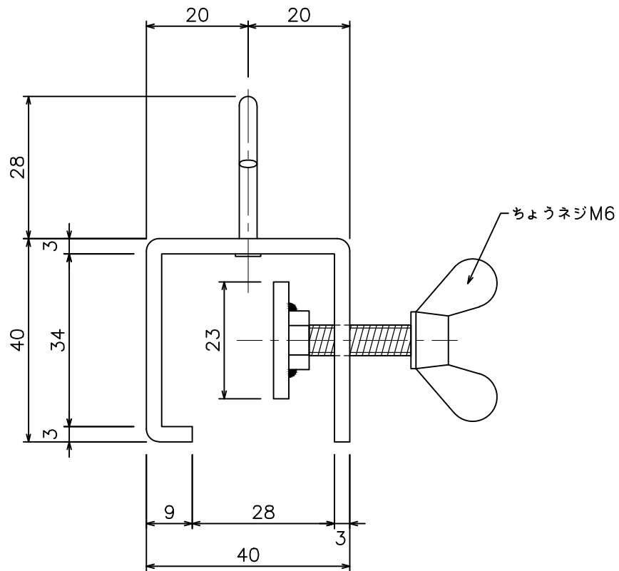
吊り金具A (15Y61)
