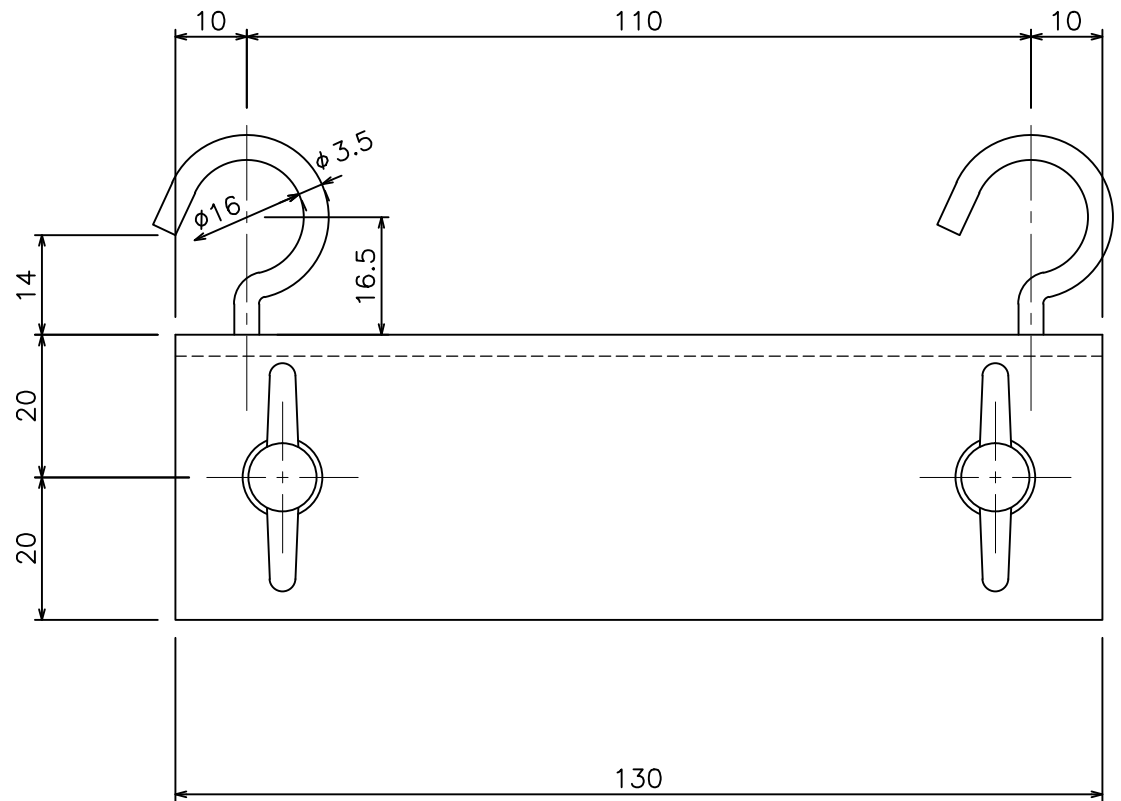
吊り金具A (15Y61)
