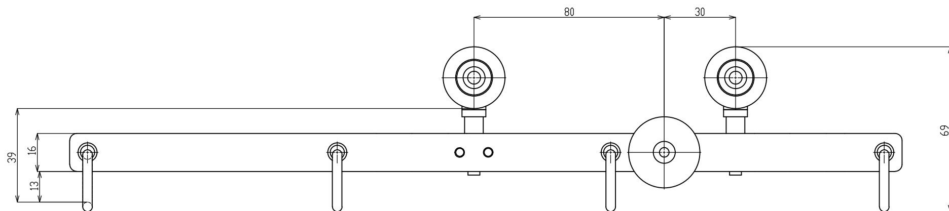
XG・MG付手引用交叉ランナー (29T69)
