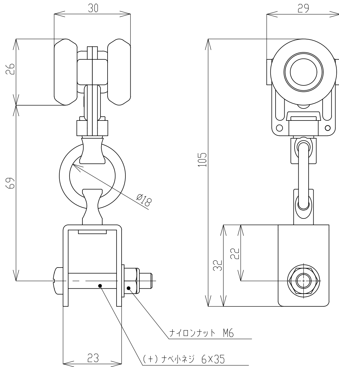
XG間仕切用ランナー (29T28)
