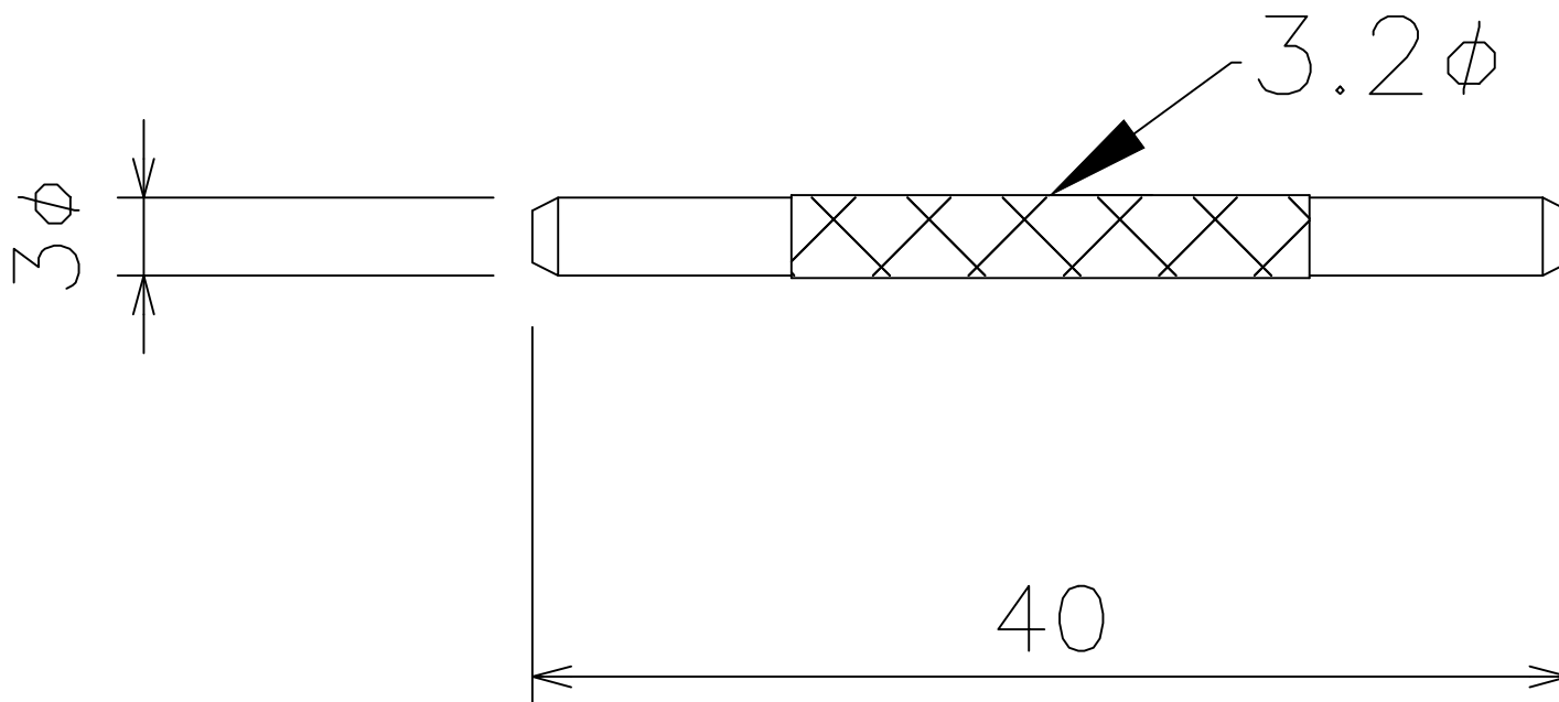
ステンローレットジョイント
